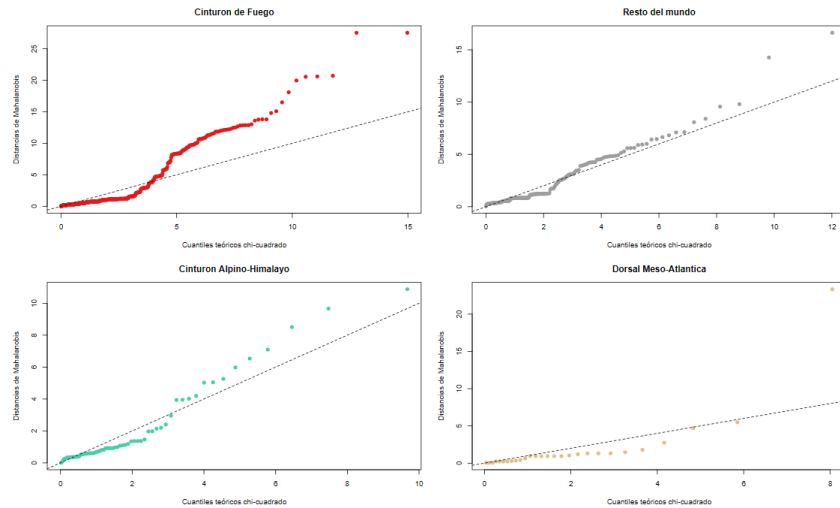
Figura 4. QQ-plots multivariantes de Mahalanobis por zona sísmica.
