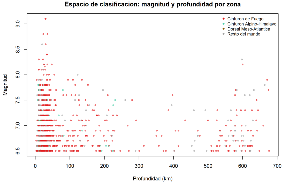
Figura 9. Espacio de clasificación: magnitud y profundidad por zona.
